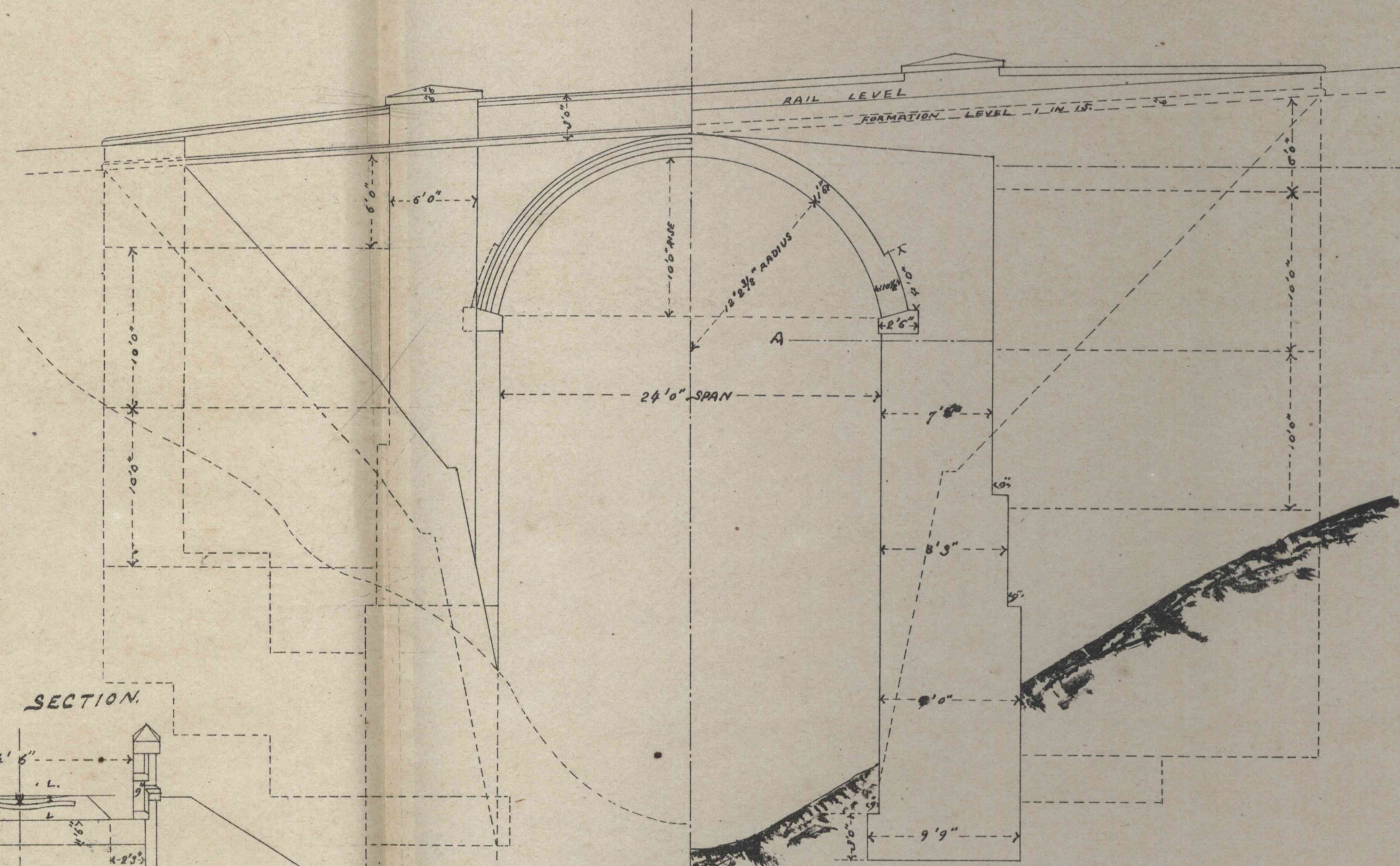
LONGITUDINAL SECTION.
