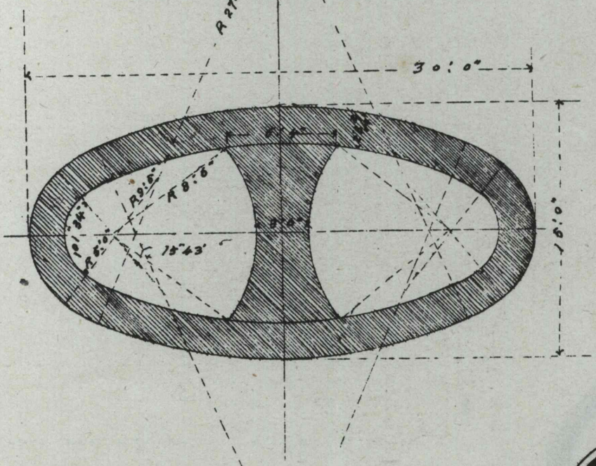
平面
