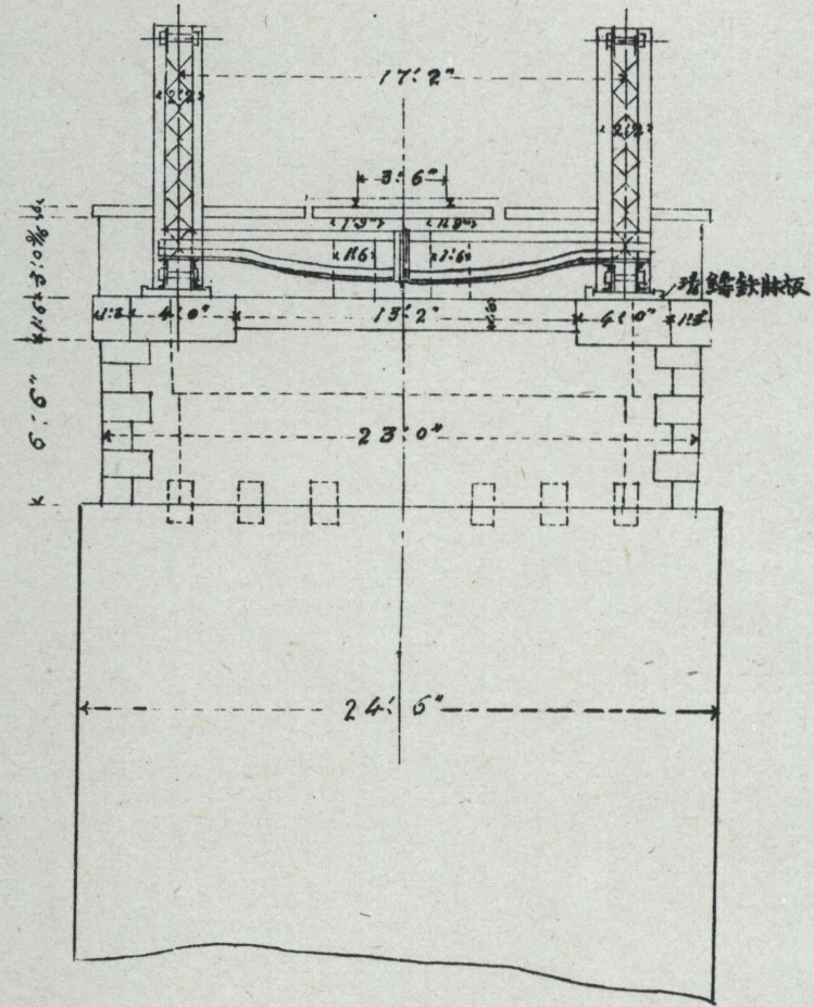
正面
