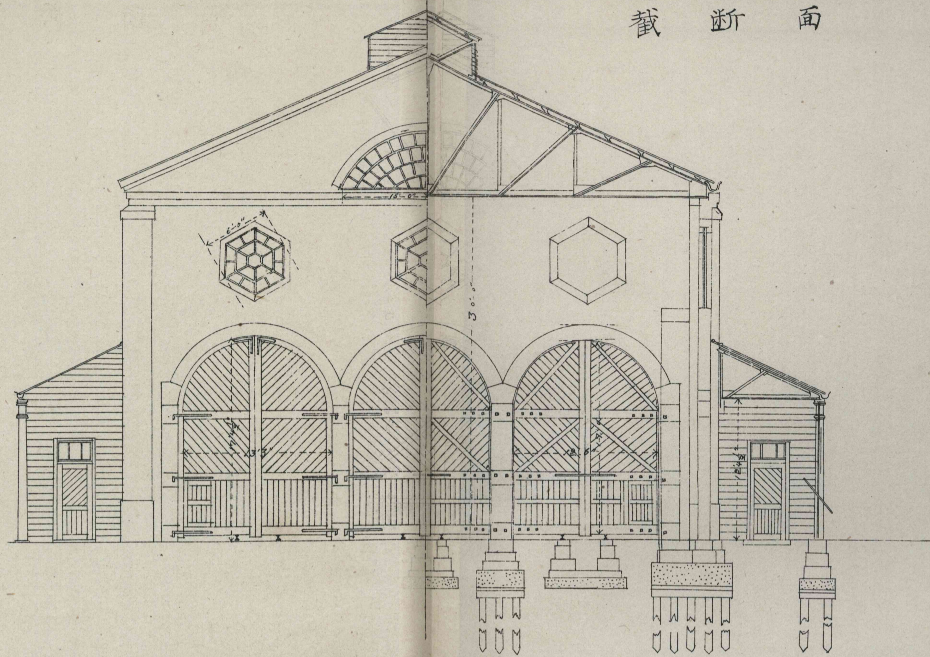
新橋停車場構内機關車修繕工場之圖 其壹
