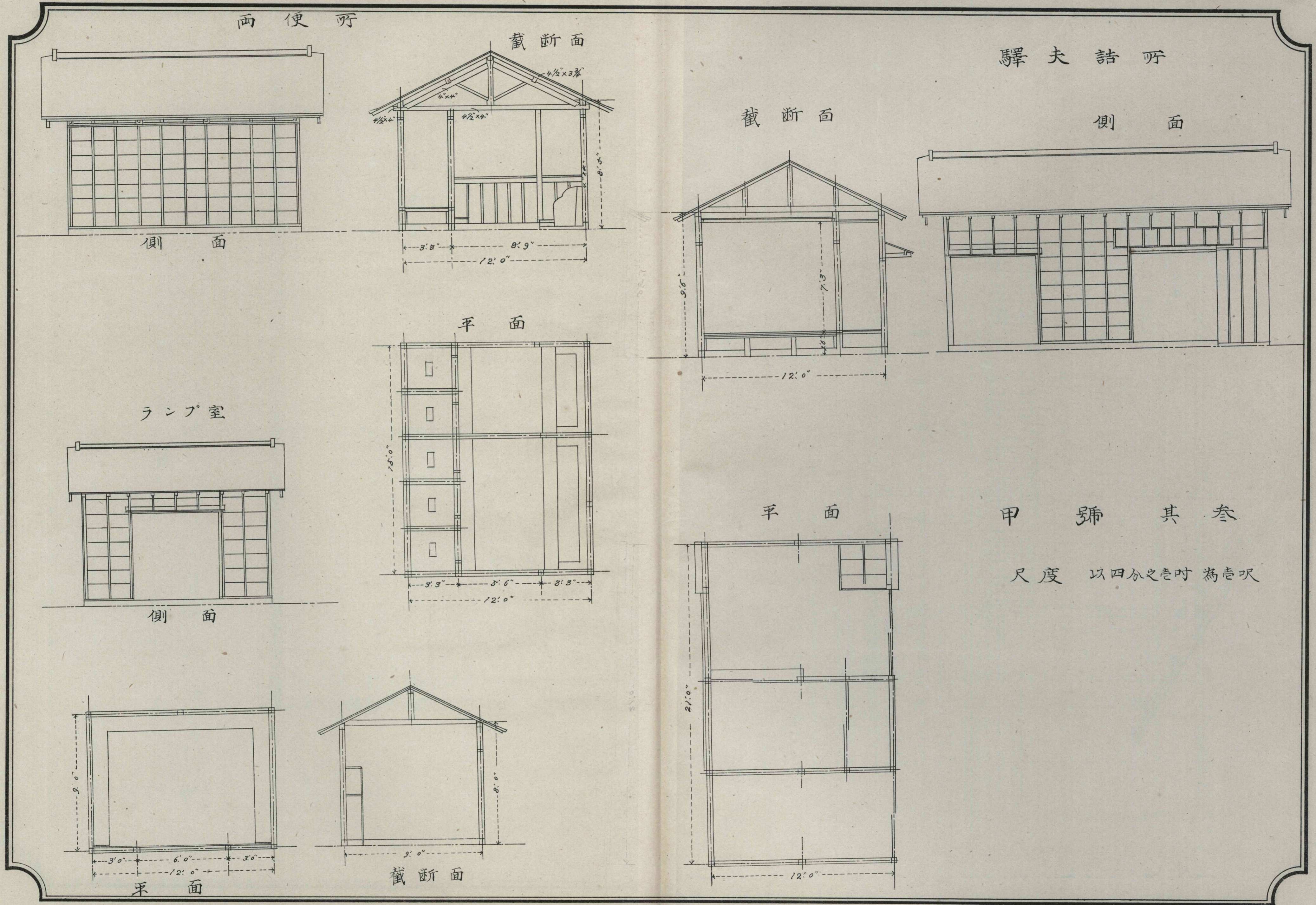
第三圖 普通停車場木屋及附屬建物ノ圖 (甲號) 共三
