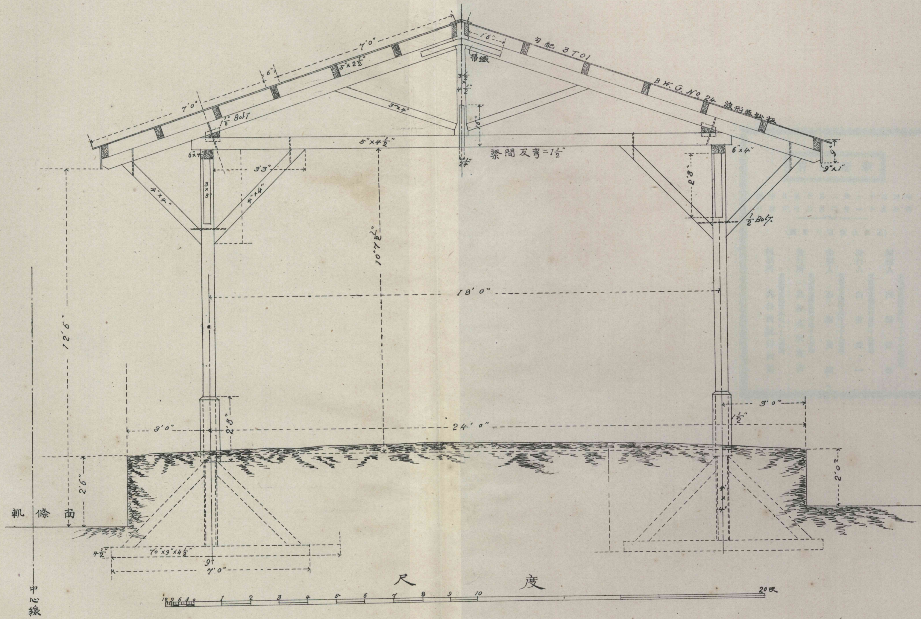
波形垂鉛葺荷物取扱所之圖
