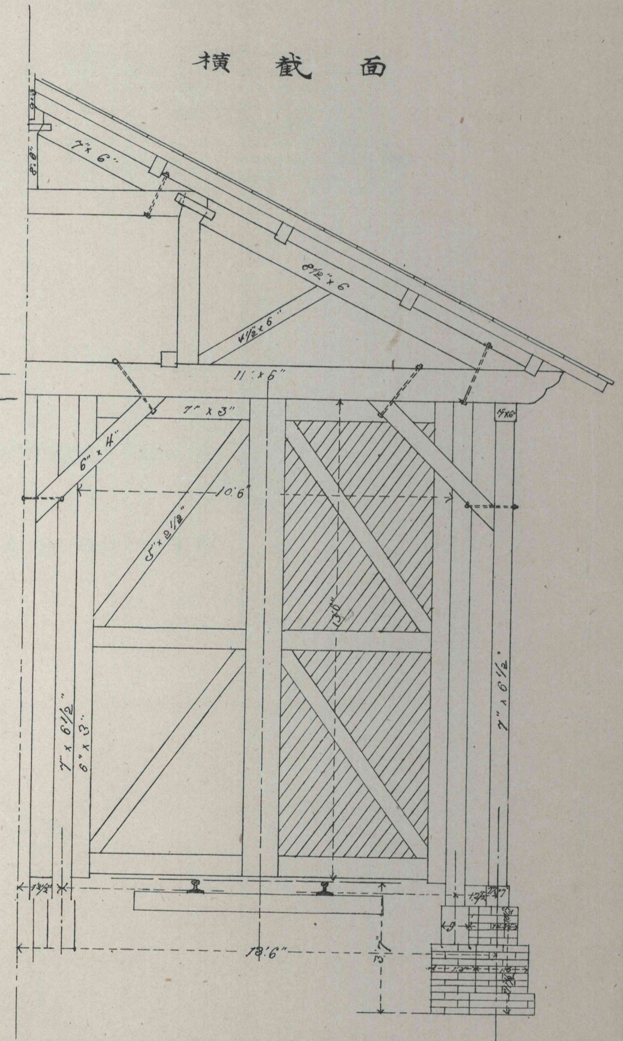
尺度 以八分三吋 爲壹呎
