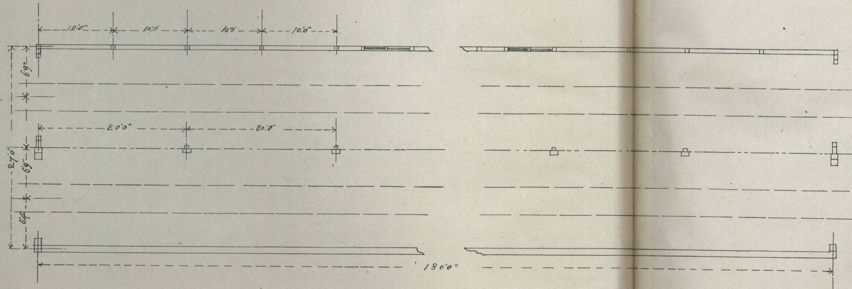
尺度 以八分三吋 爲壹呎
