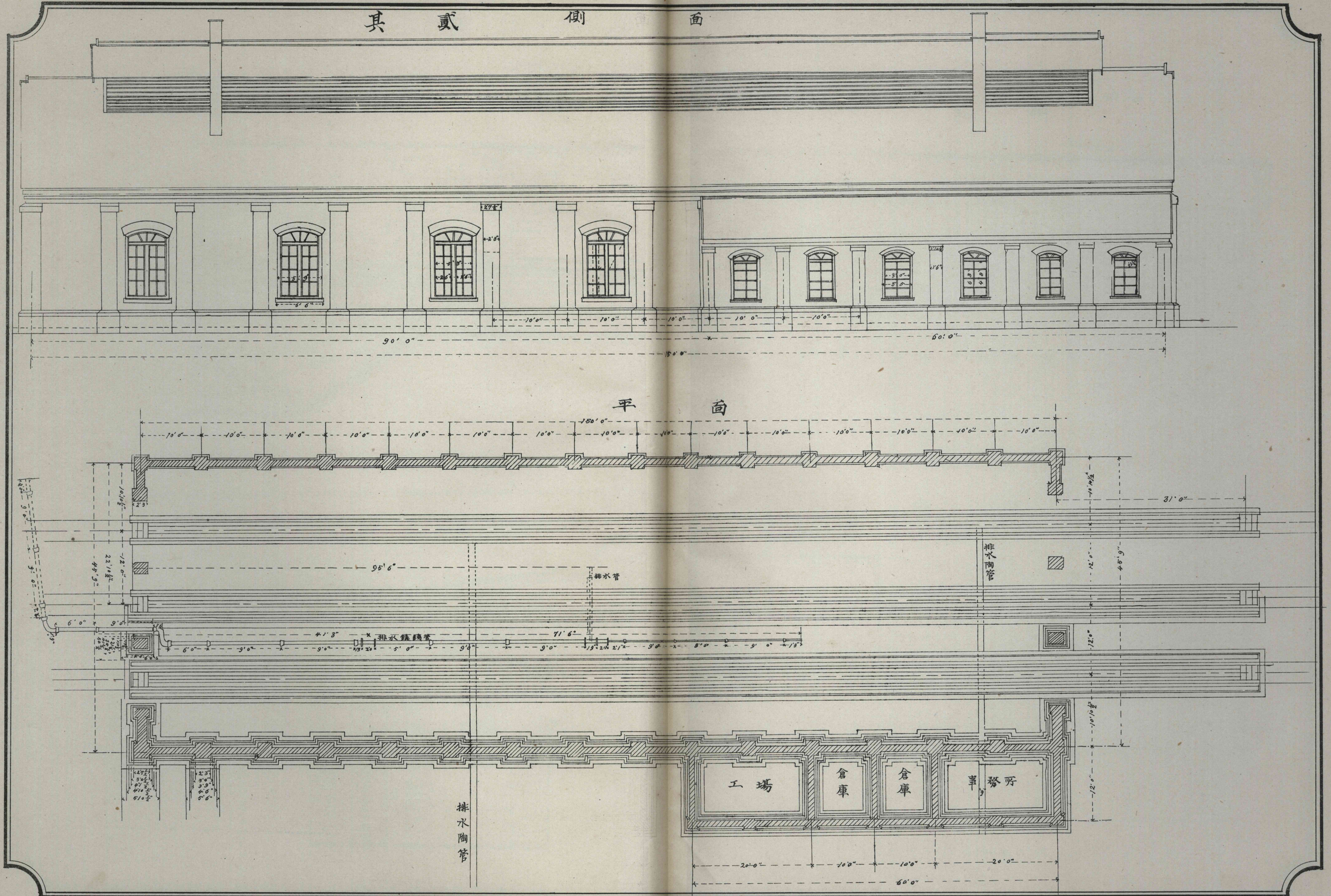
第十二圖 濱松停車場機關車庫之圖 其二
