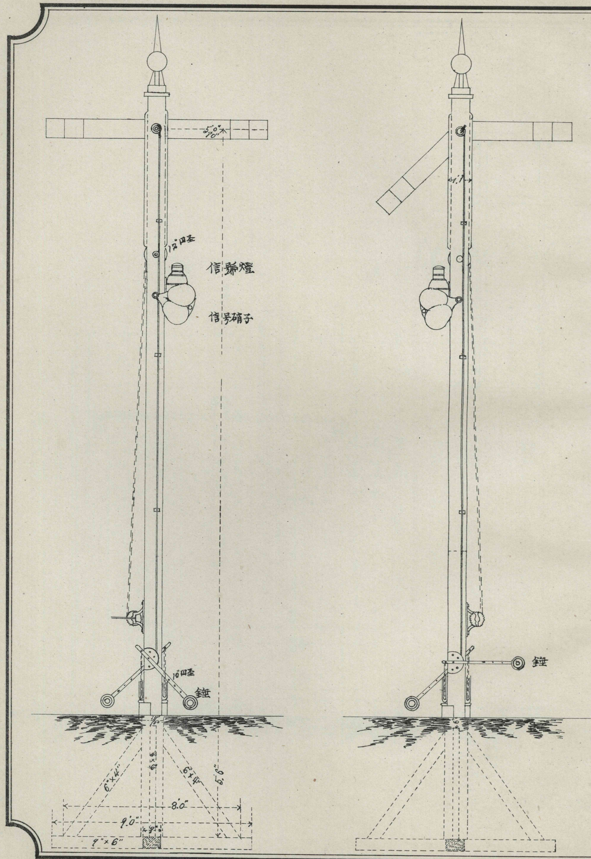
第四圖 信號機之圖
