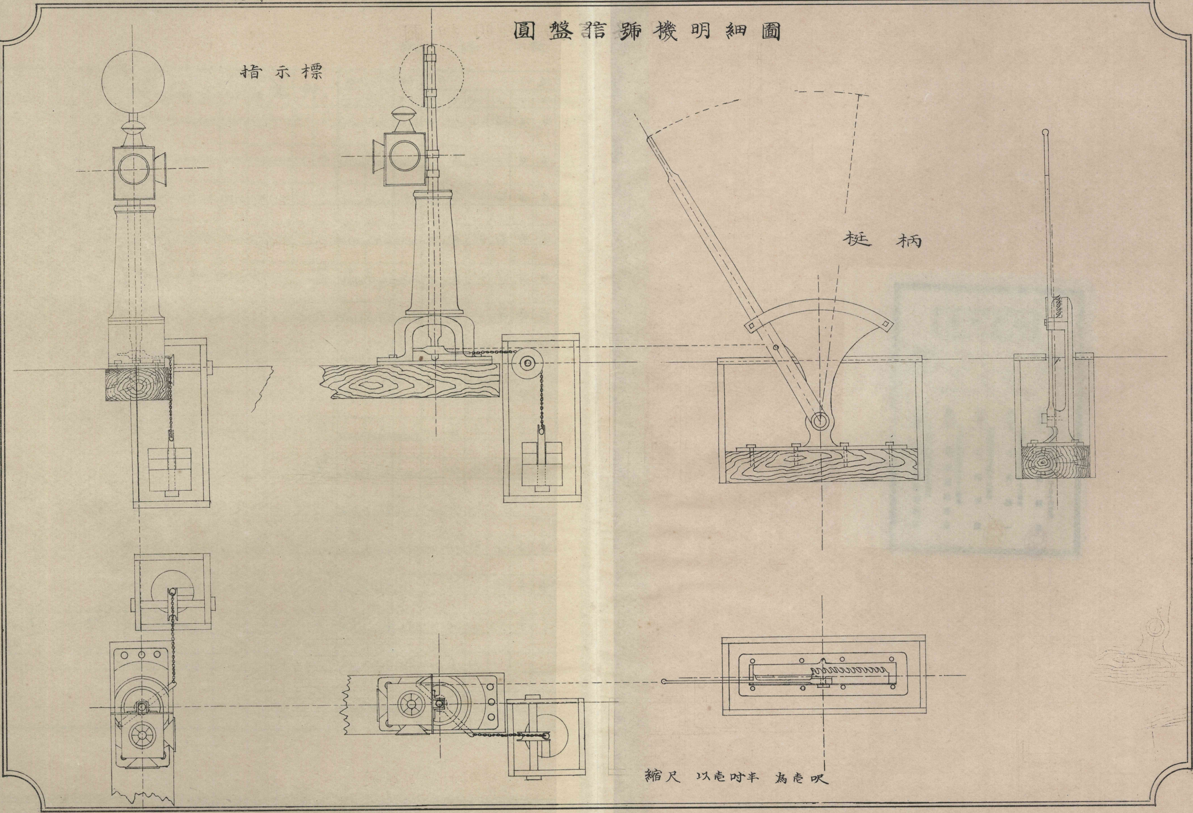
第二十圖 圓盤信號機
