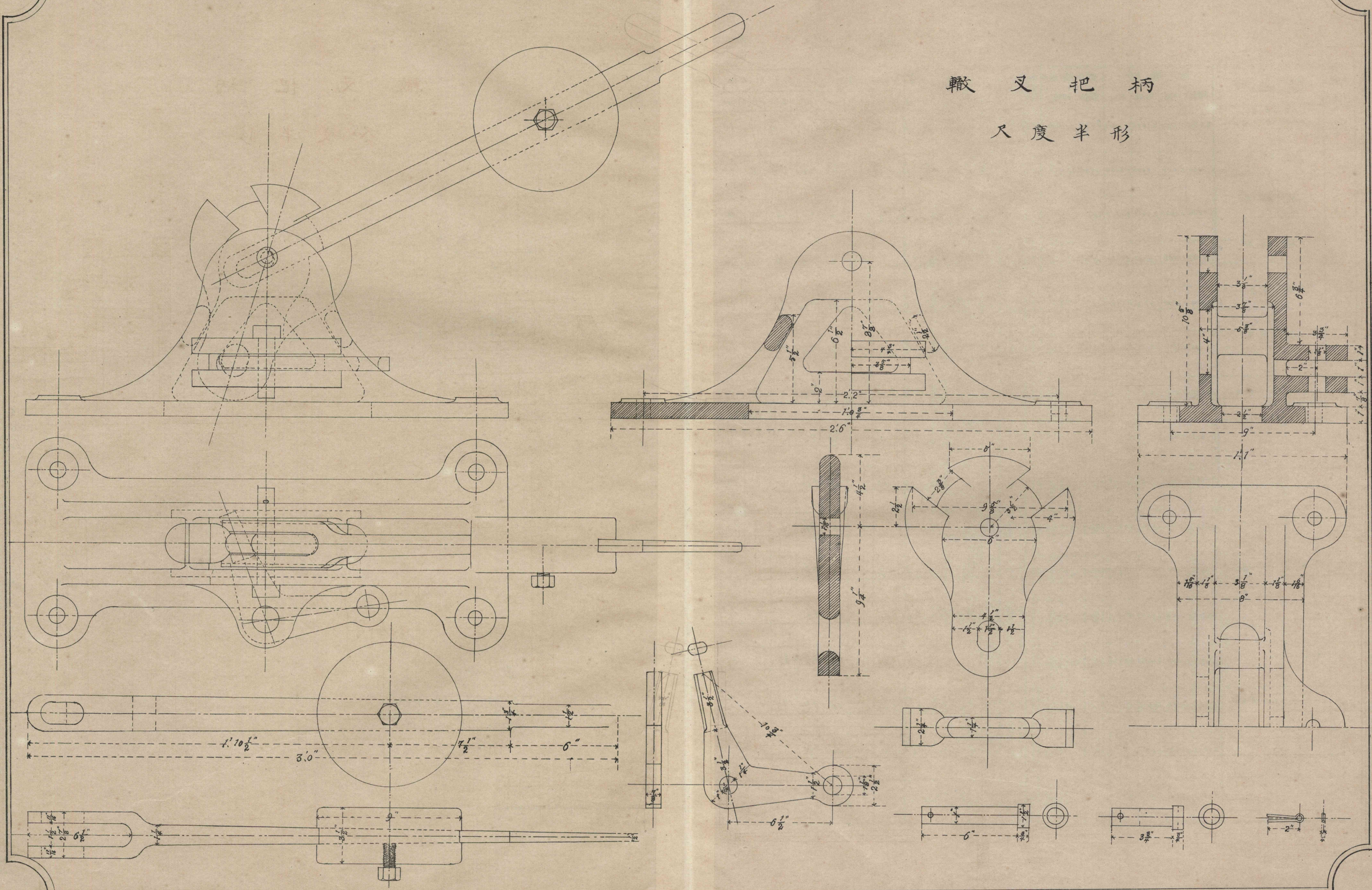
第十八圖 轆叉把柄
