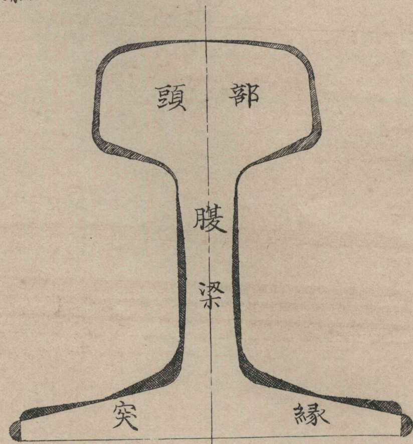
新旧軌條断面比較圖
