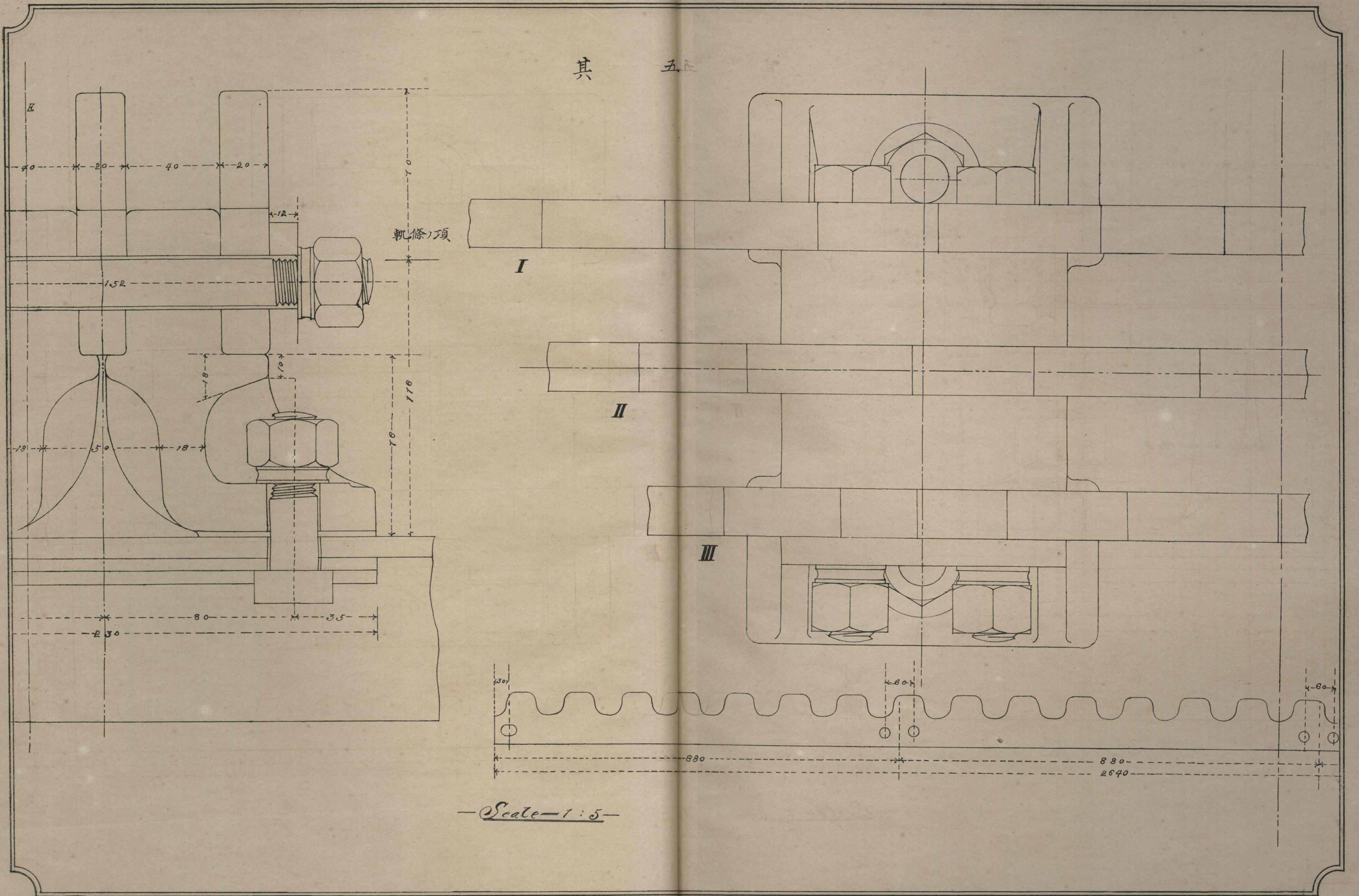
第六圖 有齒桿軌條 (アブ式) 其五
