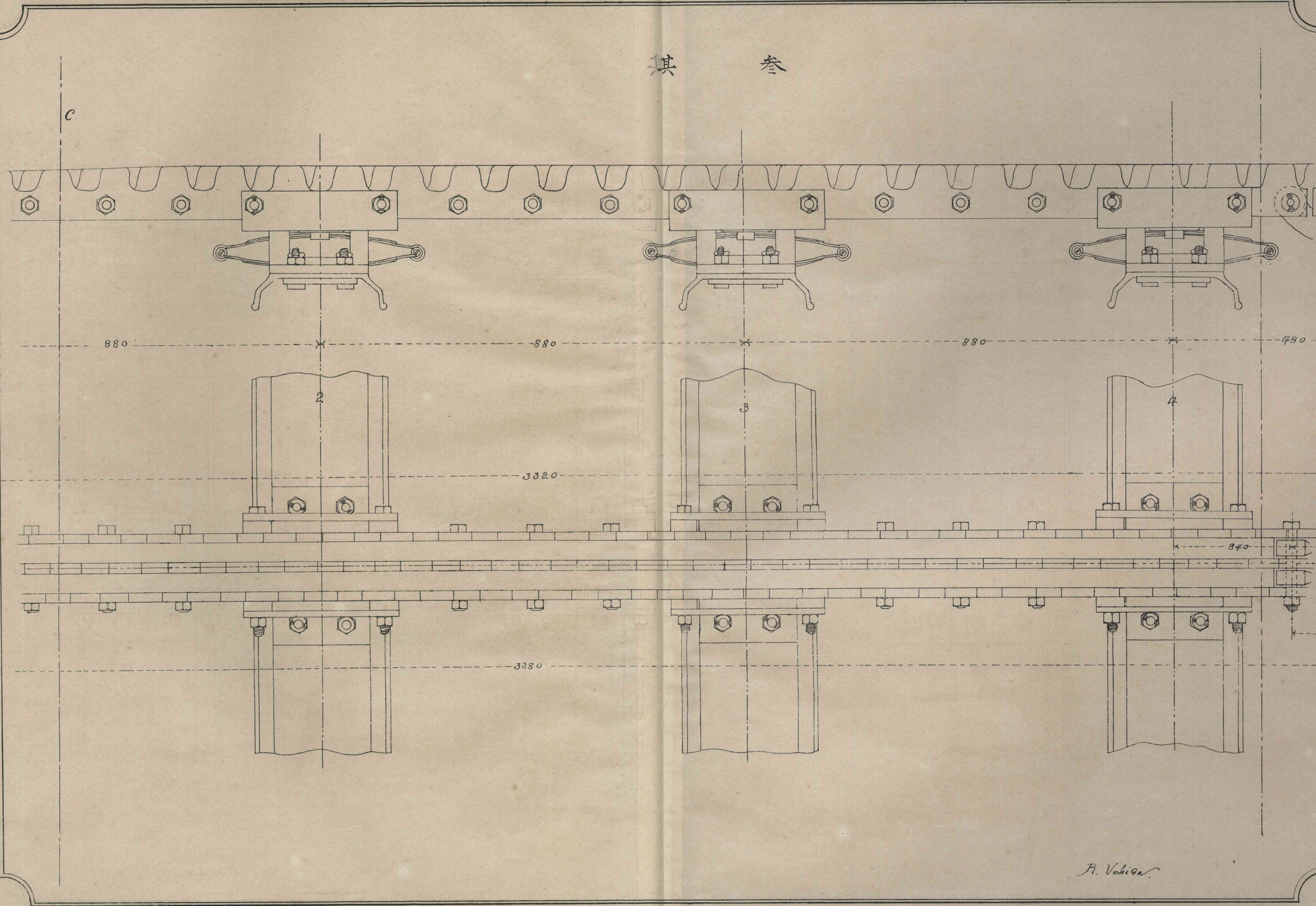
第四圖 有齒桿軌條 (A7T式) 其三
