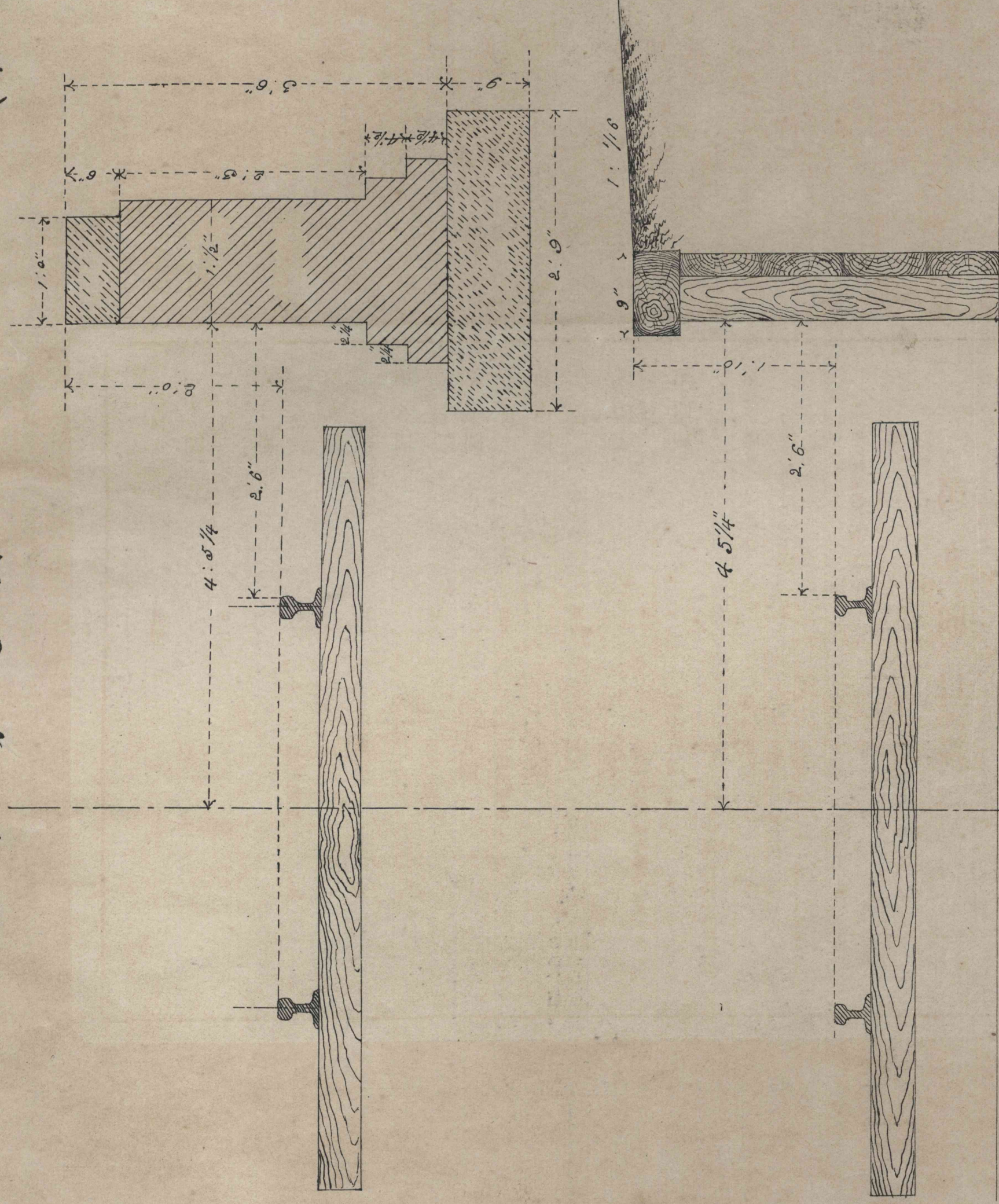
第壹圖 乘車場煉瓦造及木造武程
